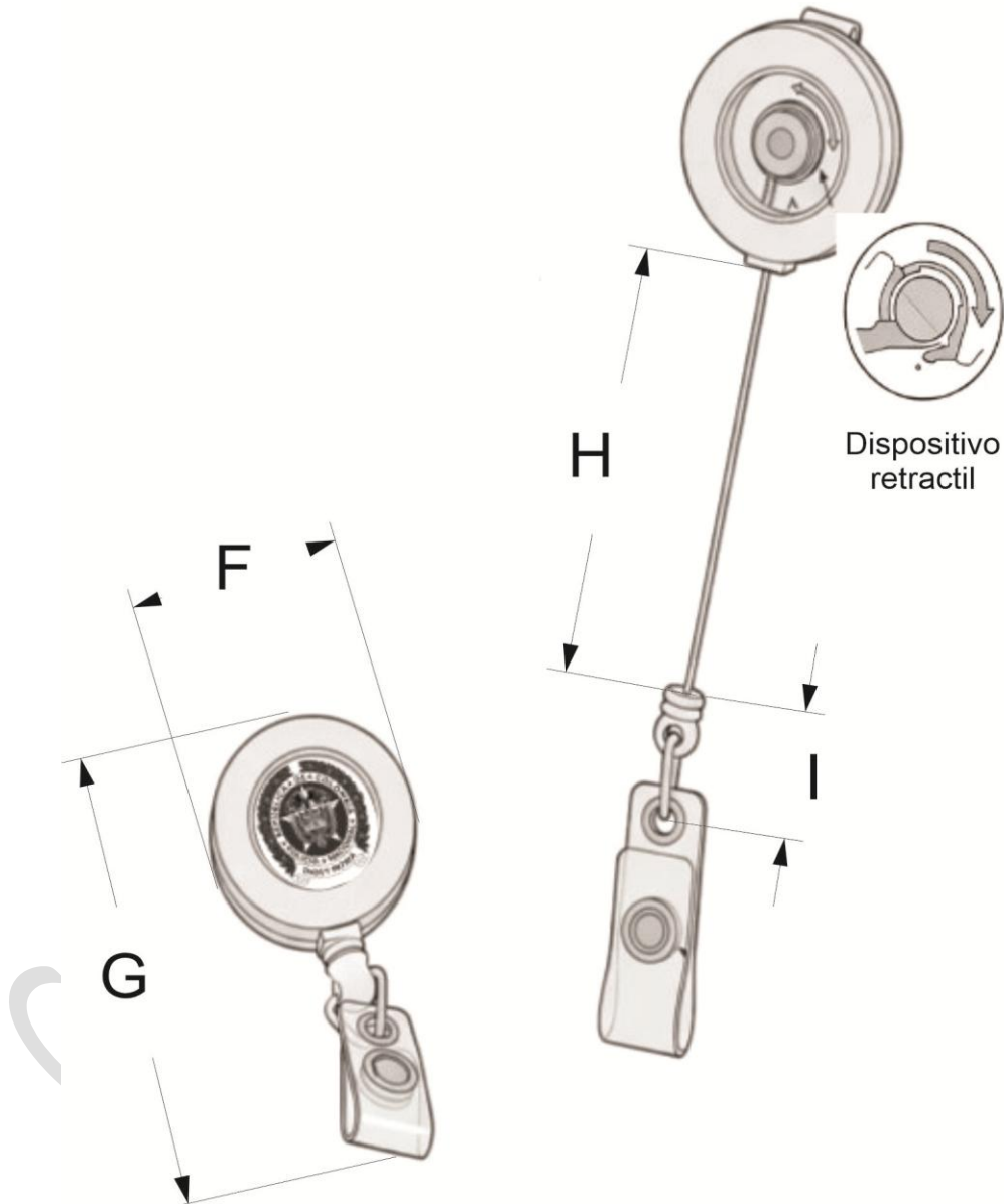
Figura 3. Dimensiones yoyo
